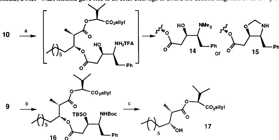
Scheme 2. Reagents: a. i) TFA / CH 2 Cl 2 ; ii) HCHO, NaBH 3 CN / MeOH ( 14 , 72%); i) TFA / CH 2 Cl 2 ; ii) HCHO, then NaBH 3 CN ( 15 , 67%). b. i) p-TsOH / MeOH (67%); ii) TBSCl, Imd / DMF (97%). c. MeI, NaH / DMF (35%)
